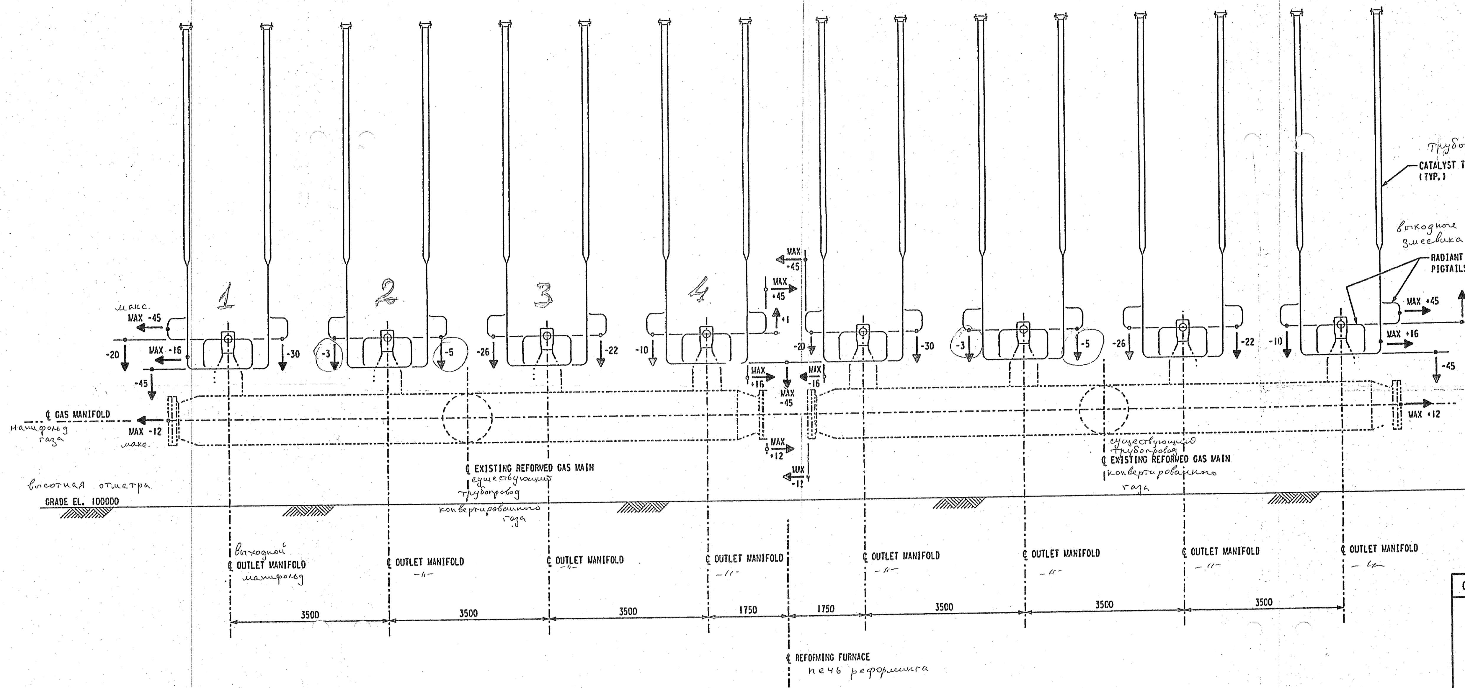
высота- движение выходного пигтейла змеевика радиальной зоны ELEVATION - RADIANT COIL OUTLET PIGTAIL MOVEMENTS
